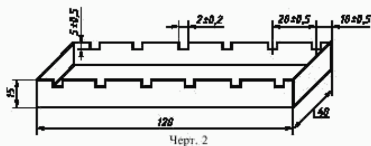
Подставка для старения образцов
