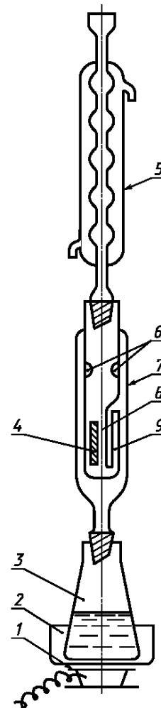
1 — электроплитка; 2 — песчаная баня; 3 — колба с n -гептаном; 4 — патрон с полимером; 5 — шариковый холодильник; 6 — отверстия; 7 — экстрактор; 8 — ловушка экстрактора; 9 — сифон
