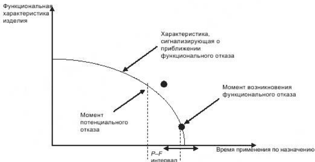
Рисунок 6 – P-F интервал
