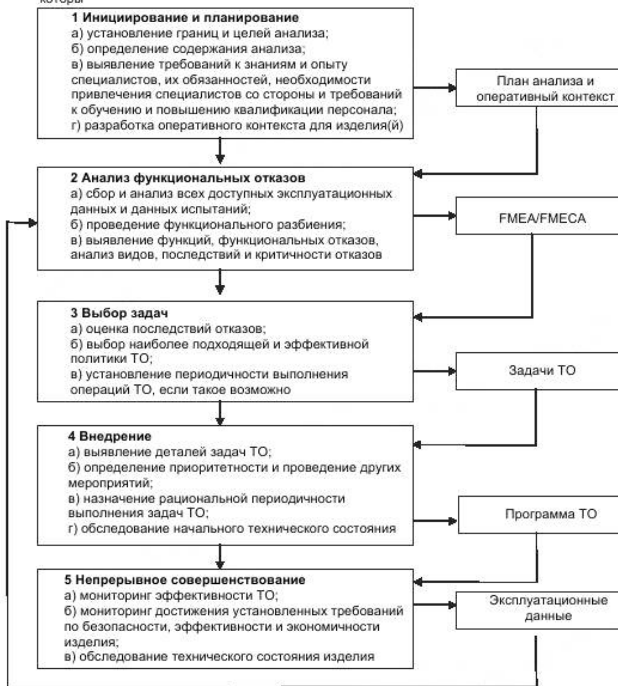
Рисунок 1 – Обзор процесса RCM
