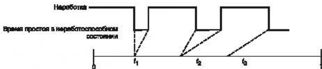
Рисунок 7 — Пример наработок между отказами одного восстанавливаемого ремонтируемого изделия
