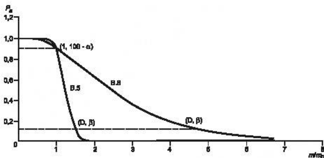
Рисунок 3 — Оперативные характеристики планов испытаний В.5 и В.8
