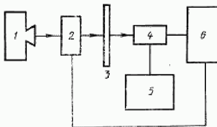
Блок-схема установки для измерения послесвечения экранов
