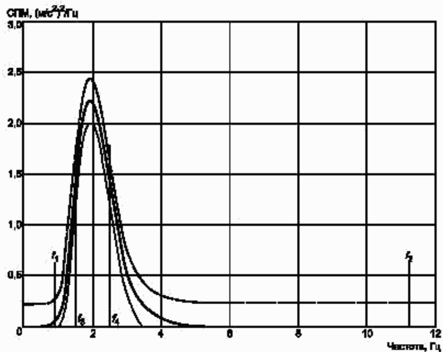
Рисунок 2 — СМВ для спектрального класса ЕМ 1 (самосвал с жесткой или шарнирно-сочлененной рамой снаряженной массой более 4500 кг)
