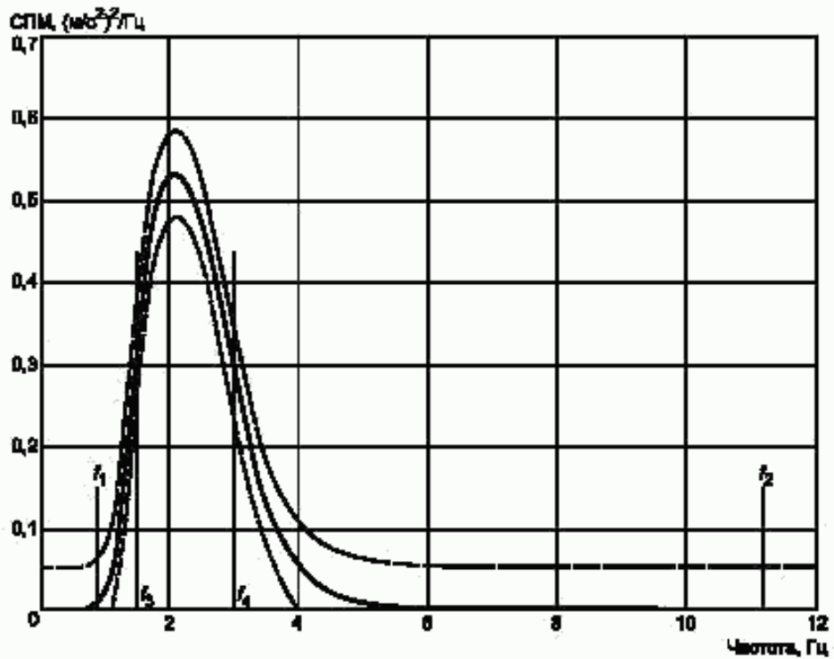
Рисунок 5 — СПМ для спектрального класса EM 4 (грейдеры)
