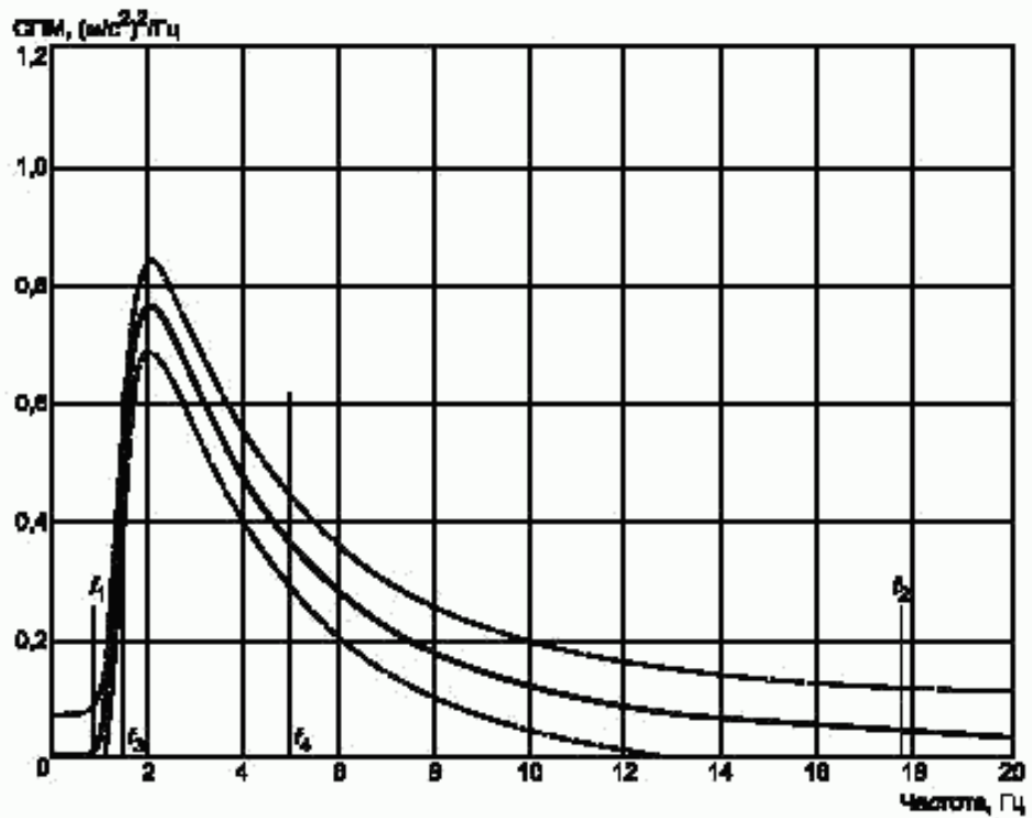
Рисунок 6 — СПМ для спектрального класса EM 5 (колесные бульдозеры, колесные катки, погрузчики с обратной лопатой)
