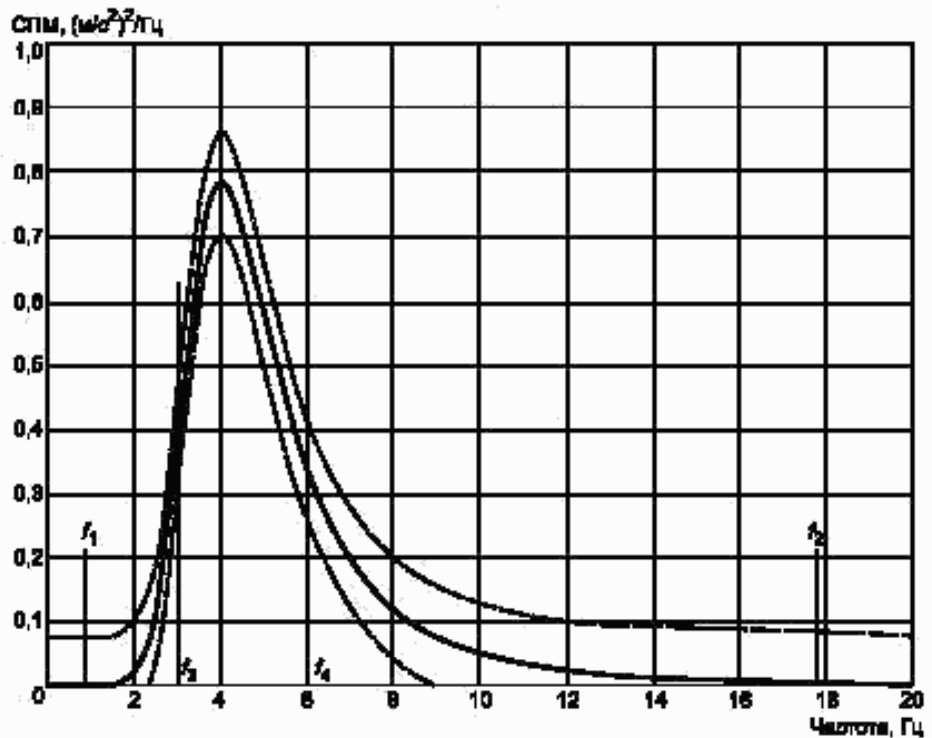
Рисунок 10 — СПМ для спектрального класса EM 9 (погрузчики с бортовым поворотом массой менее 4500 кг)
