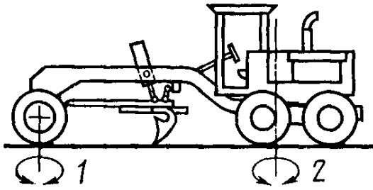
1 — управляемые колеса; 2 — центр поворота
