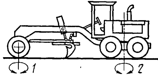
1 — управляемые колеса; 2 — центр поворота
