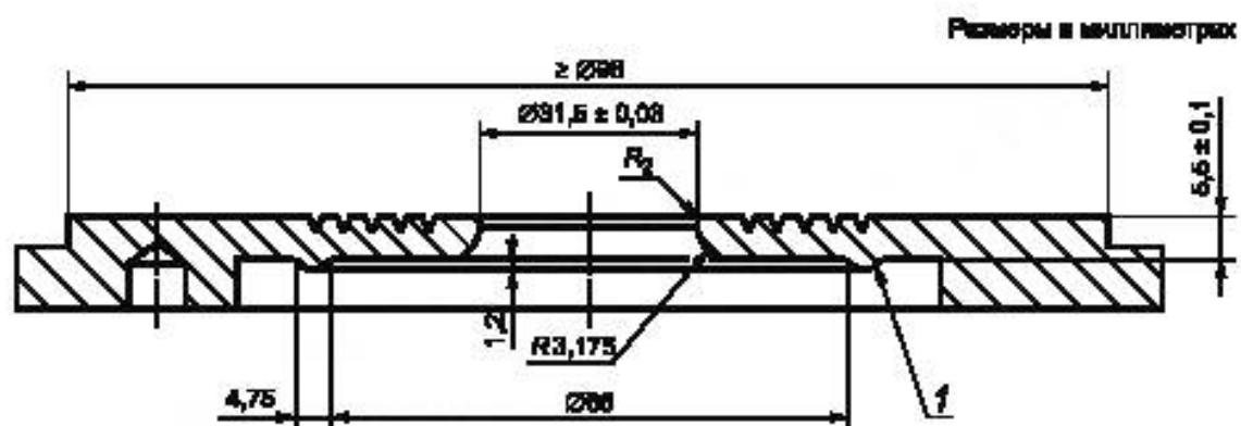
Рисунок А.2 — Вариант нижнего зажима
