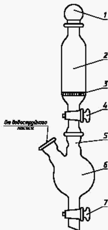
1 — пробка (притертая); 2 — фильтрующая делительная воронка; 3 — впаиваемый стеклянный фильтр № 2 или 3; 4, 7 — сливные краны; 5 — соединительный шифр; 6 — приемник экстракта
