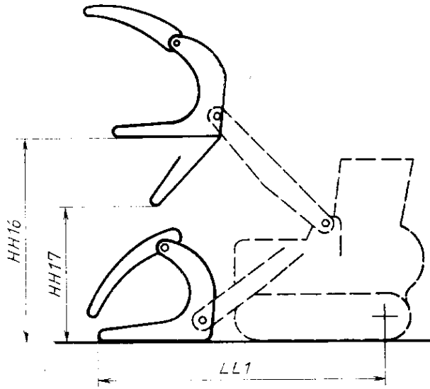
Черт. 22. Размеры челюстного захвата
