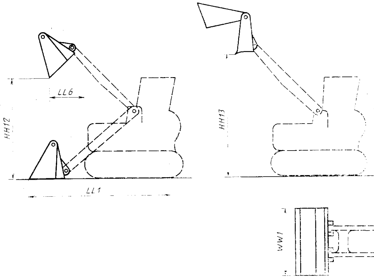
Черт. 20. Размеры двухчелюстного ковша
