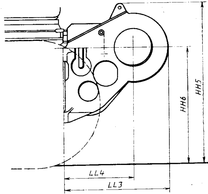
Черт. 23 Размеры лебедки
