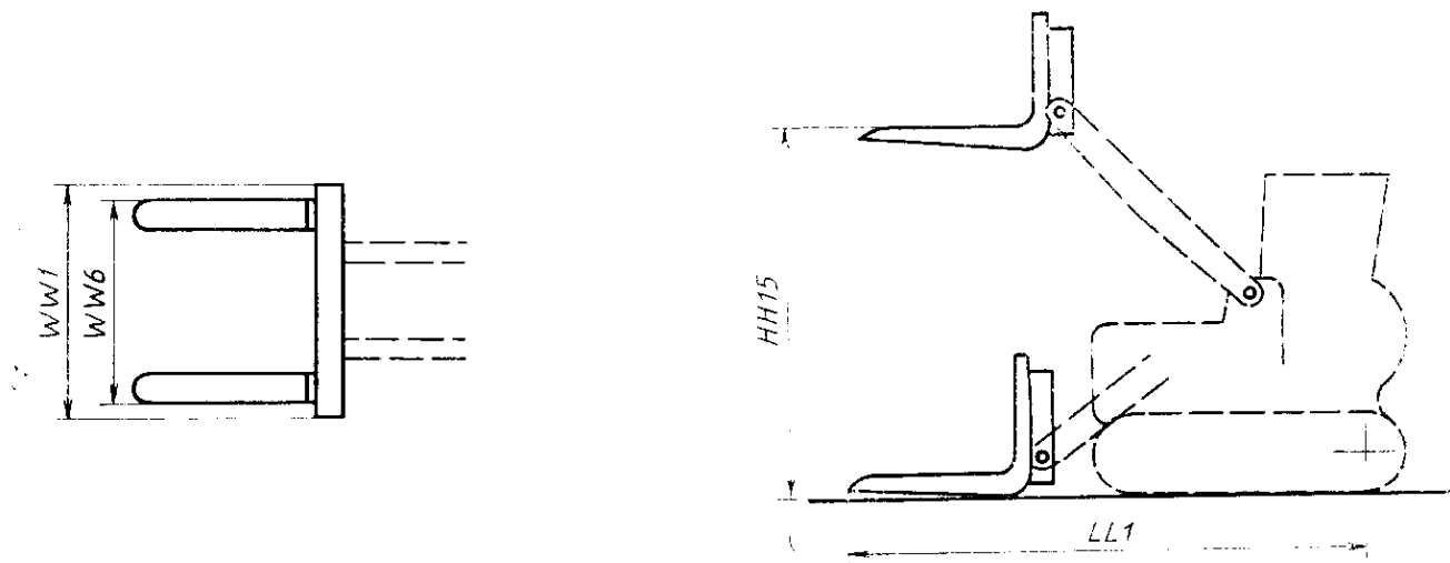
Черт. 21 Размеры грузовых вил
