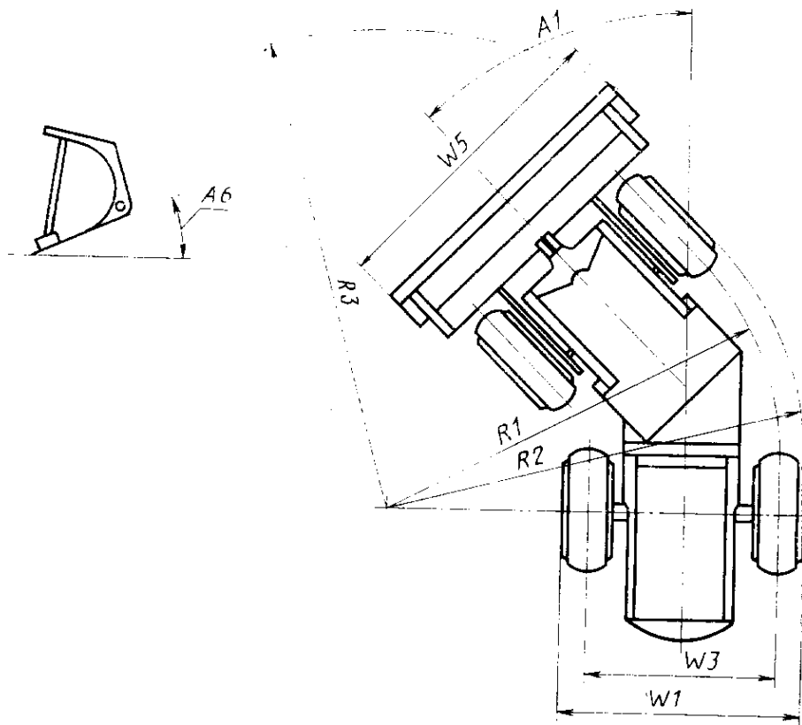
Черт. 16. Размеры базовой машины (колесного погрузчика)
