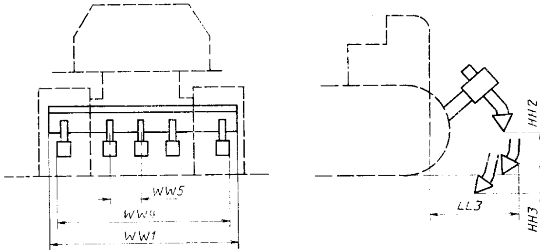
Черт. 18. Размеры рыхлителя
