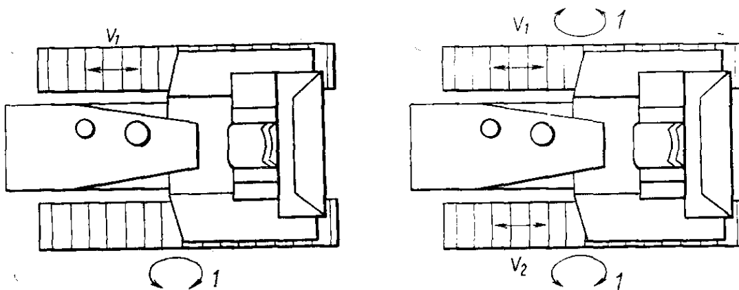
Черт. 11. С независимым вращением движителей каждого борта, v_1 \neq v_2 (гусеничный погрузчик)
