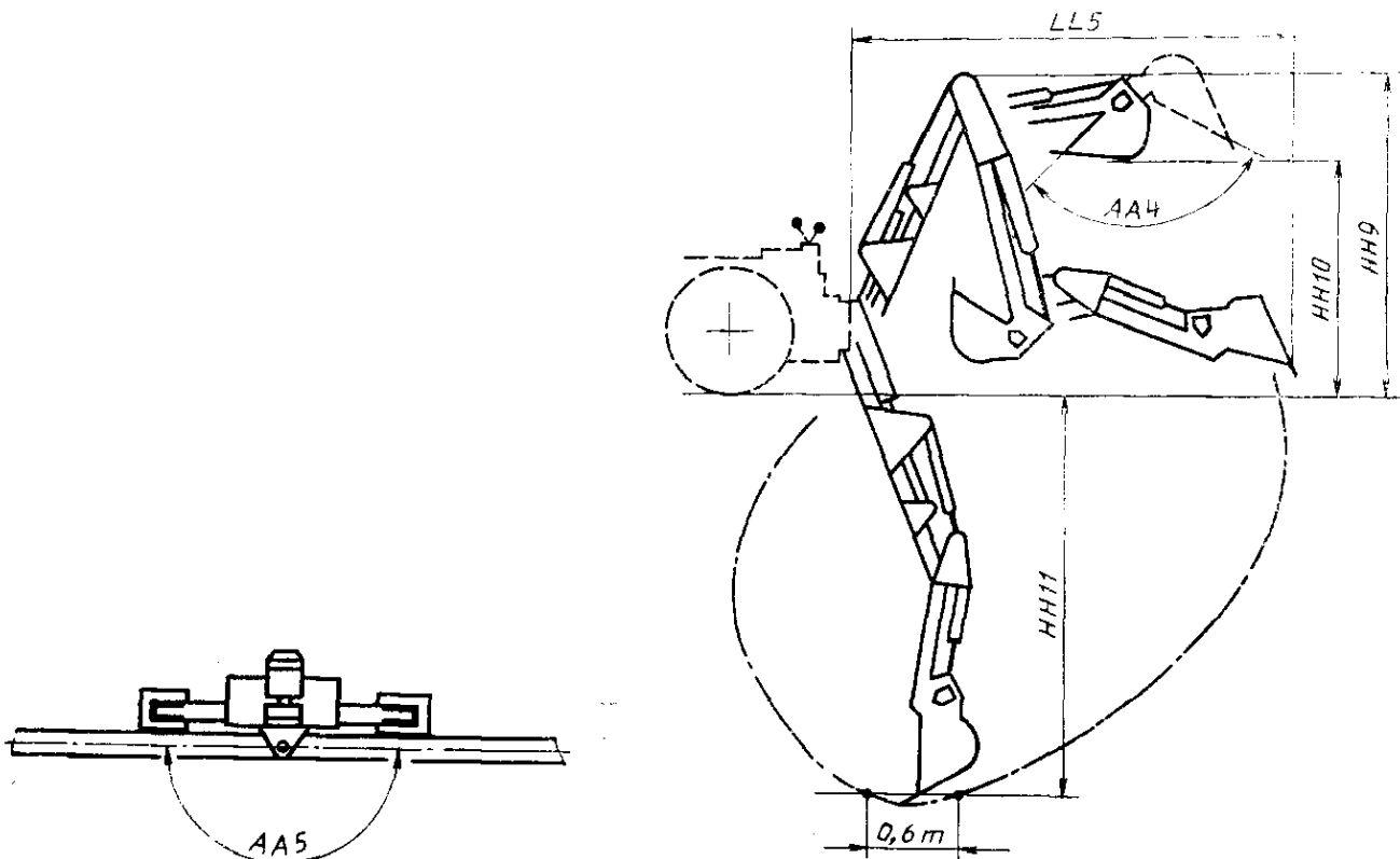
Черт. 17. Размеры обратной лопаты
