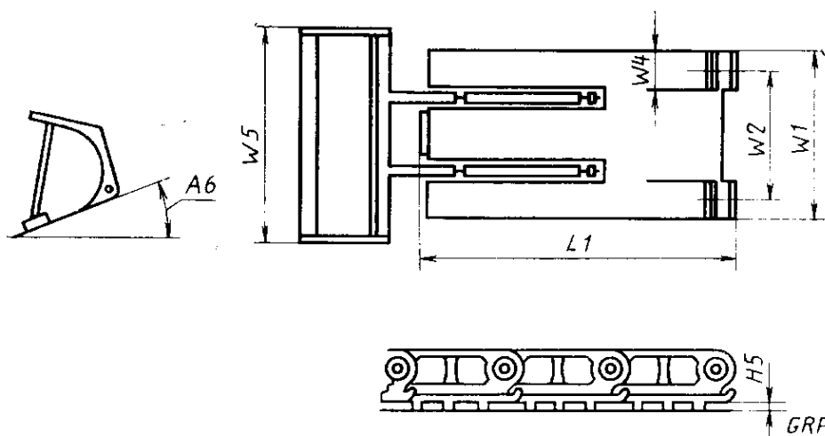
Черт. 15. Размеры базовой машины (гусеничный погрузчик)
