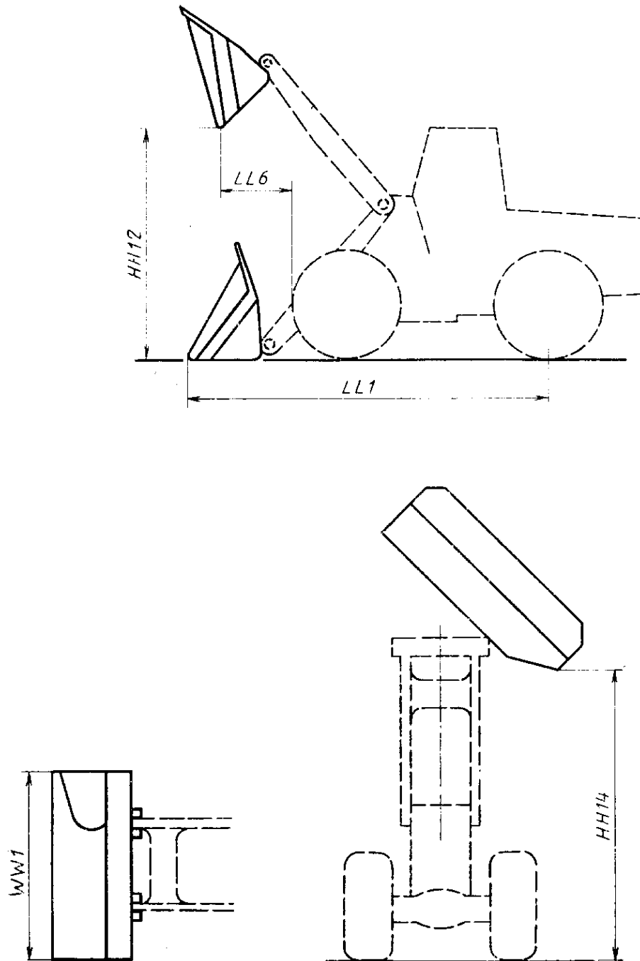
Черт. 19 Размеры ковша с боковой разгрузкой
