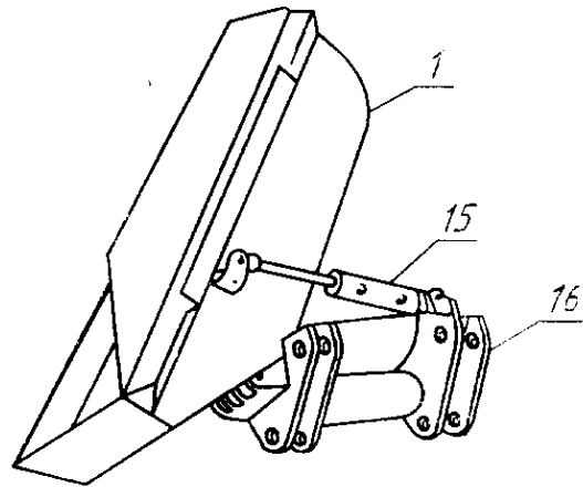
1—ковш; 15—гидроцилиндр боковой разгрузкой; 16—рама ковша с люлькой
