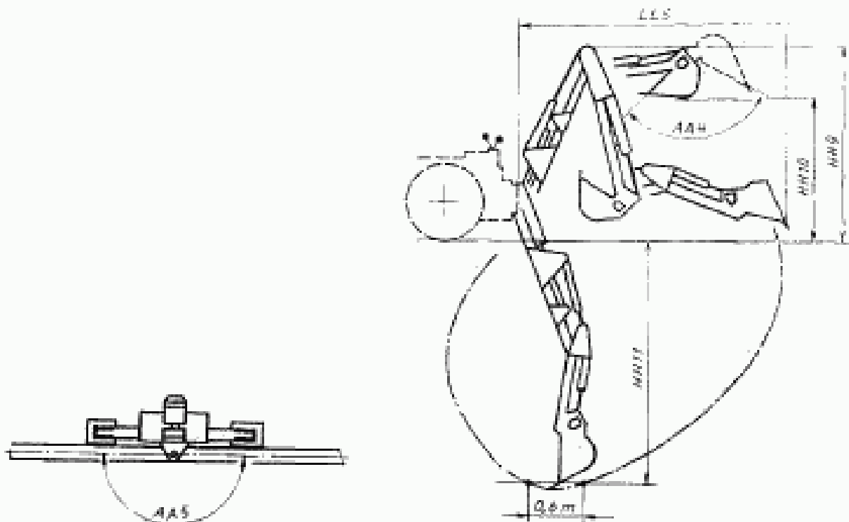
Черт. 17. Размеры обратной лопаты
