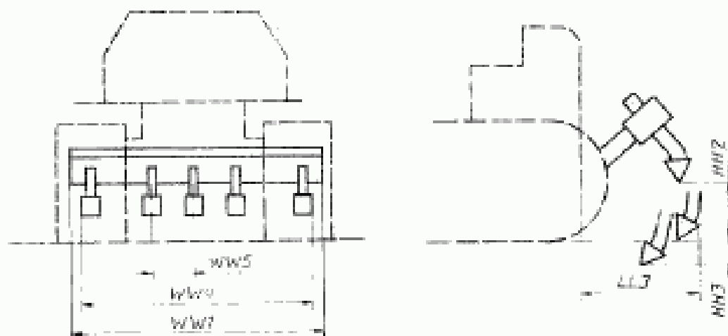
Черт. 18. Размеры рыхлителя
