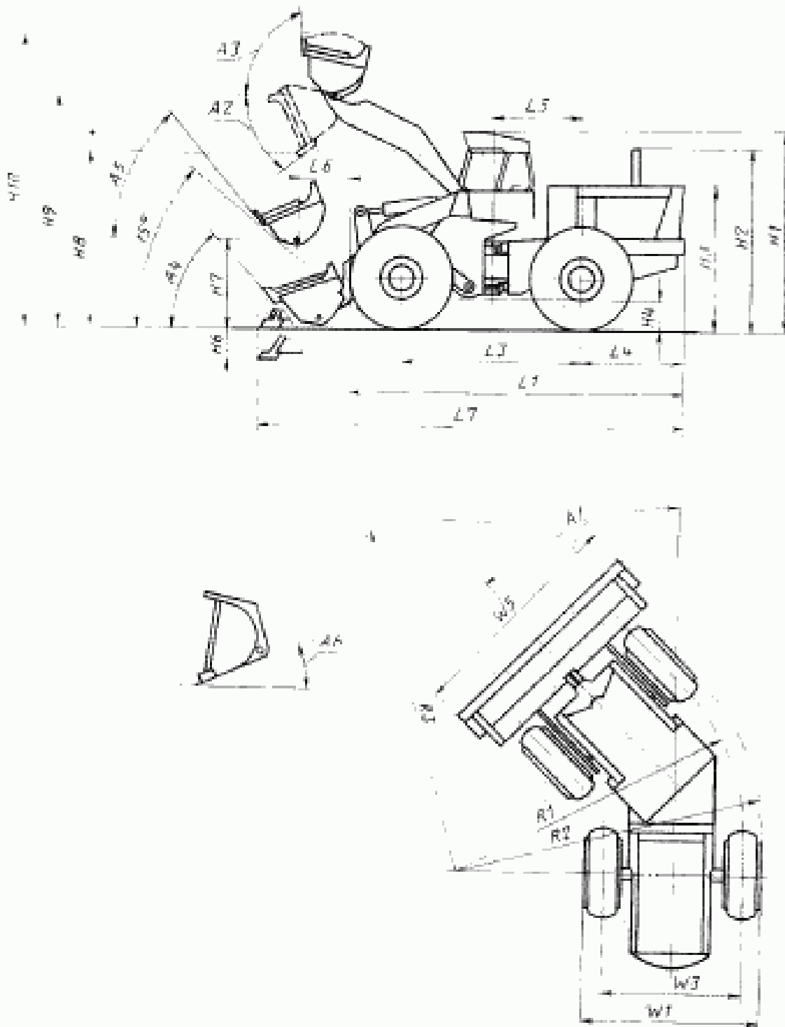
Черт. 16. Размеры базовой машины (колесного погрузчика)
