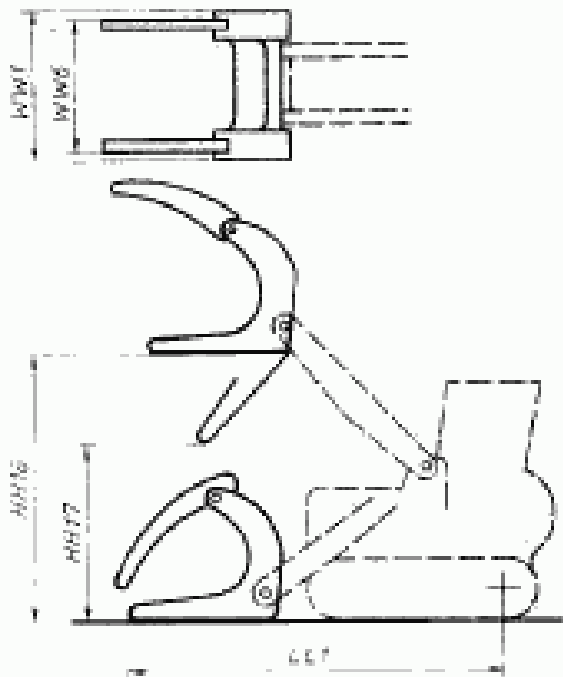
Черт. 22. Размеры челюстного захвата
