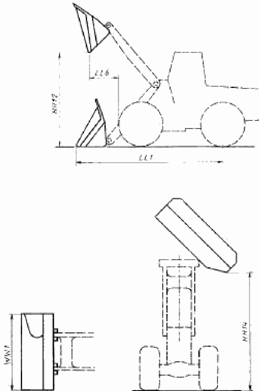
Черт. 19 Размеры ковша с боковой разгрузкой
