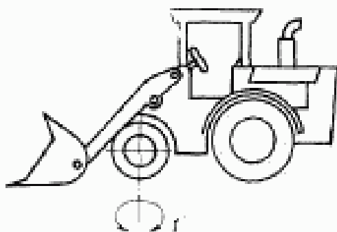
Черт. 5. С передними управляемыми колесами
