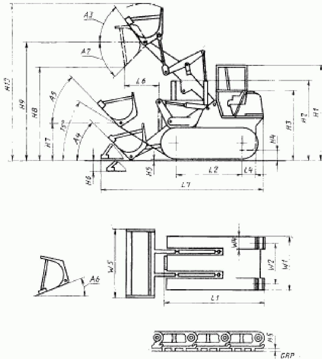
Черт. 15. Размеры базовой машины (гусеничный погрузчик)
