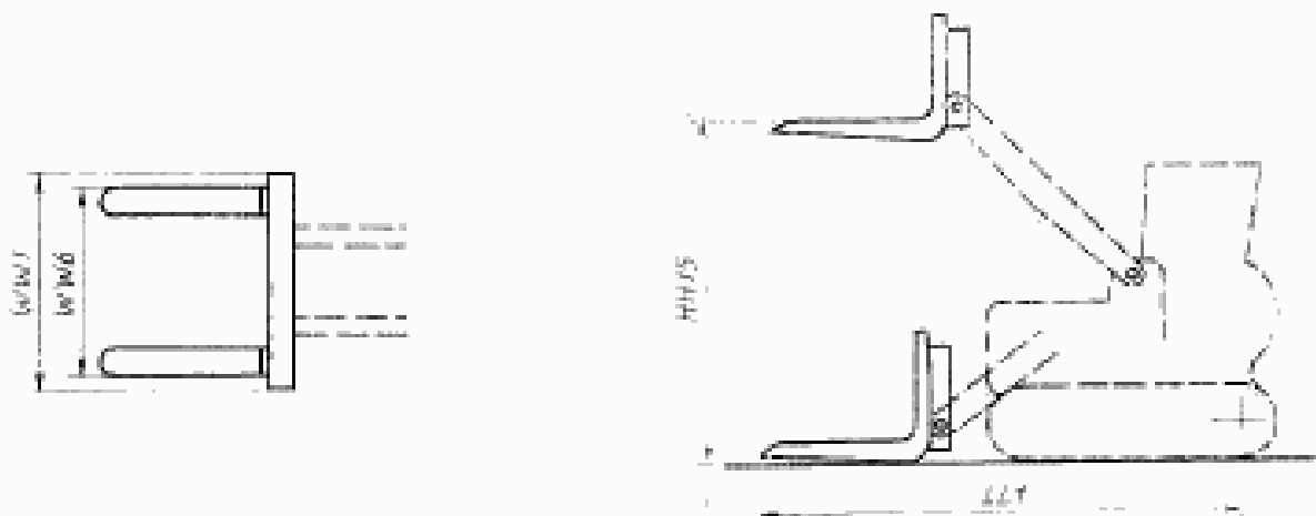
Черт. 21 Размеры грузовых вилок
