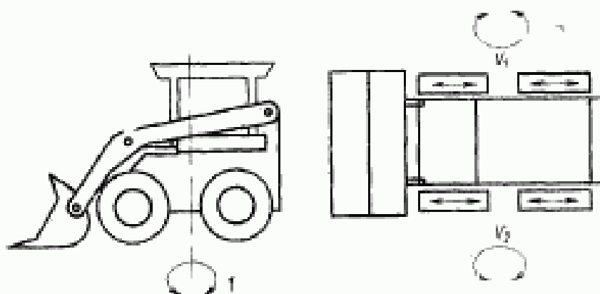
Черт. 9б. С независимым вращением двигателей каждого борта, v_1 \neq v_2 (колесный погрузчик)
