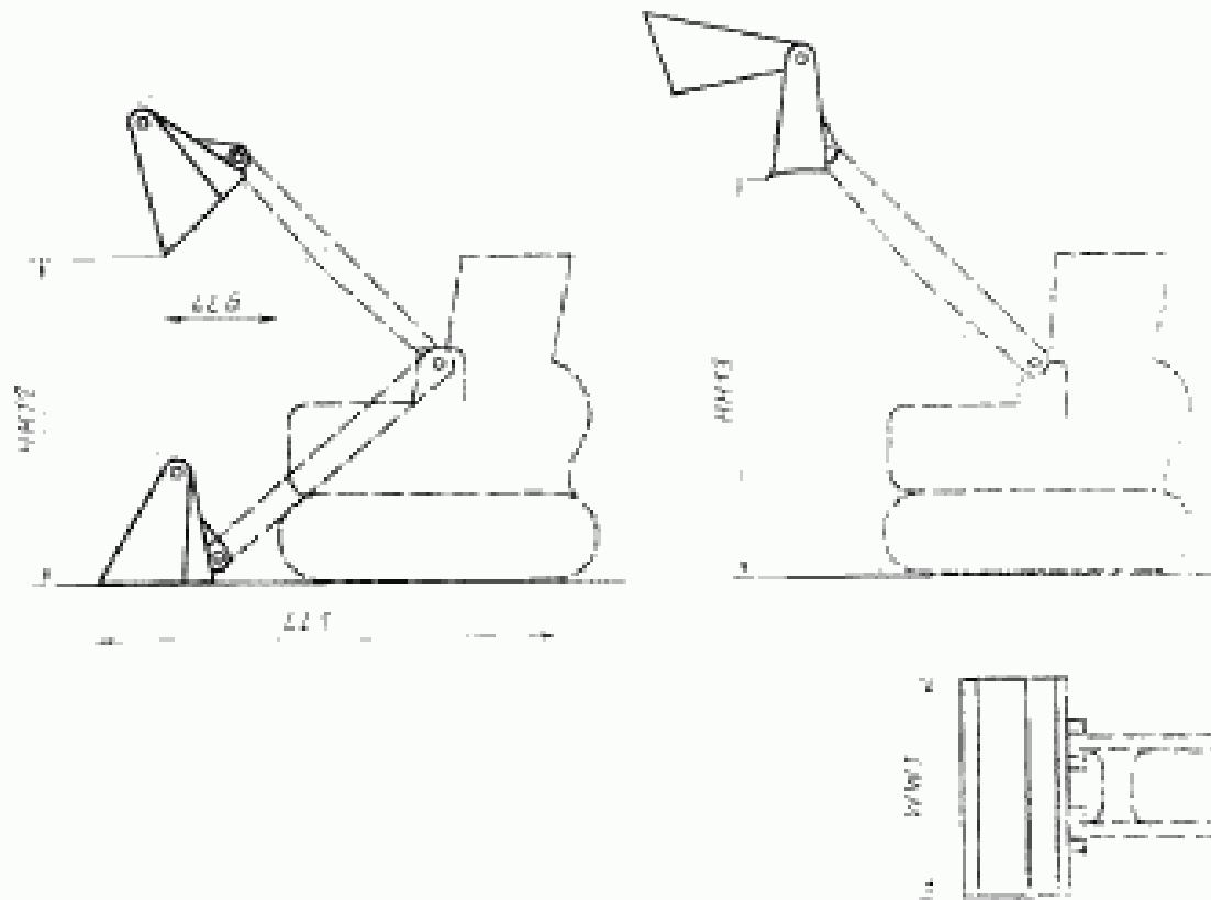
Черт. 20. Размеры двухчелюстного ковша
