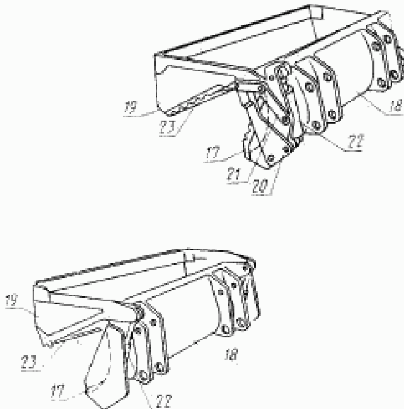
17—режущая кромка бульдозерной (нижней) челюсти; 18—бульдозерная (нижняя) челюсть; 19—верхняя (подающая) челюсть; 20—шарнир; 21—тяга верхней челюсти; 22—гидроцилиндр открывания челюсти; 23—режущая кромка верхней челюсти
