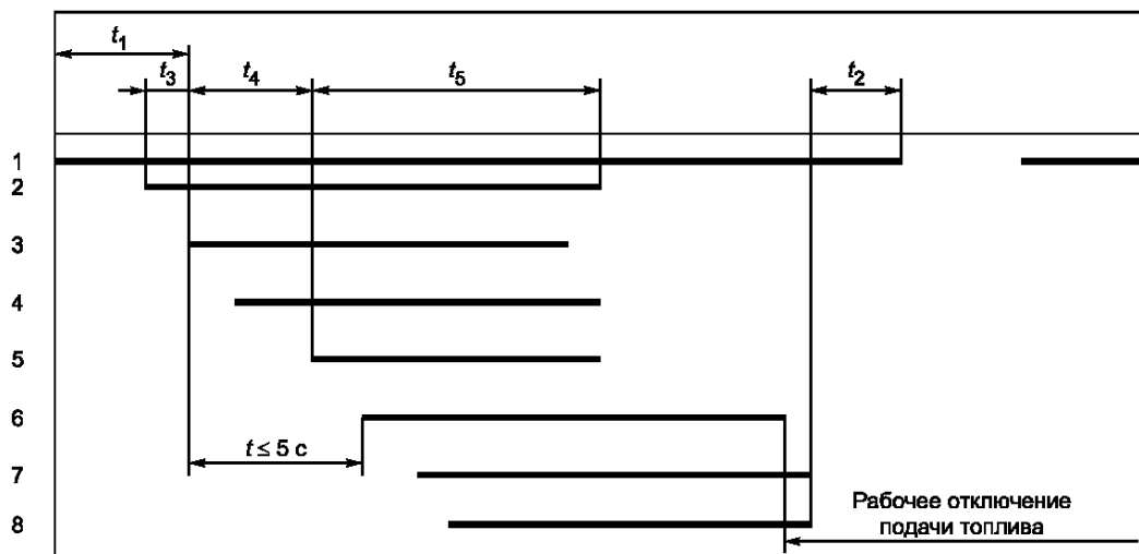
Диаграмма нормальной работы горелки
