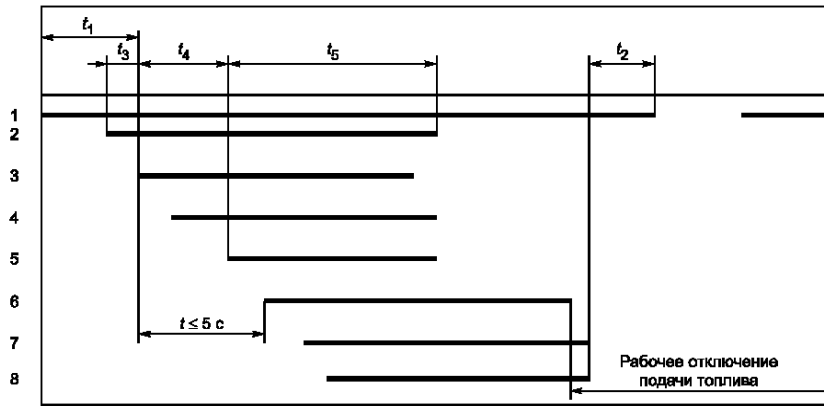
Диаграммы с защитным отключением при пуске
