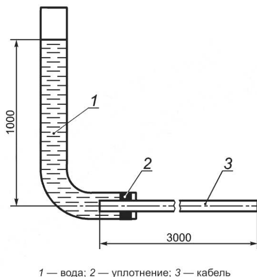
Рисунок 5 — Испытательное устройство
