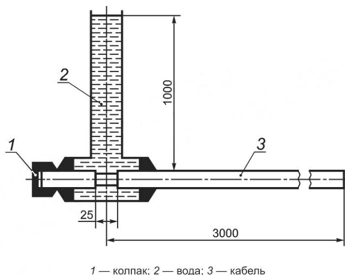
Рисунок 4 — Испытательное устройство
