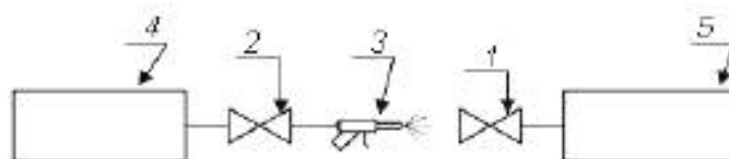
1 – испытуемый клапан, 2 – клапан, 3 – обдуватель, 4 – резервуар с пробным газом, 5 – система течеискателя
