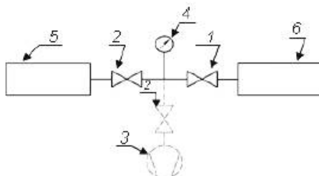
1 – испытуемый клапан, 2 – клапан, 3 – дополнительный вакуумный насос, 4 – вакуумметр, 5 – резервуар с пробным газом, 6 – течейскаатель
