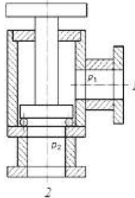
1 – полость А, 2 – полость В
