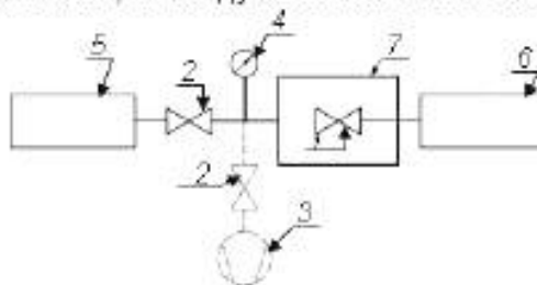
1 – испытуемый клапан, 2 – клапан, 3 – дополнительный вакуумный насос, 4 – вакуумметр, 5 – резервуар с пробным газом, 6 – система течеискателя, 7 – испытательная камера
