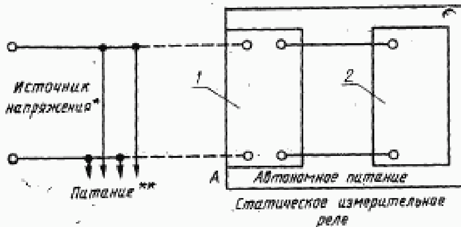
1 — вспомогательный источник реле (входной интерфейс); 2 — статические цепи
