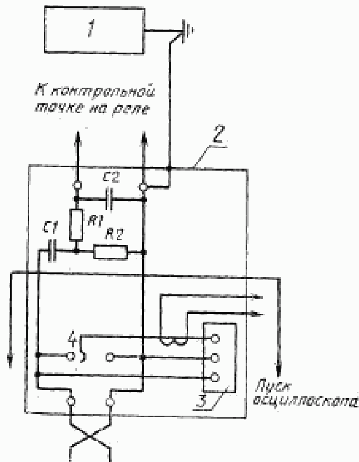
Схема импульсного генератора
