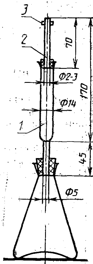
1 — стеклянная трубка диаметром 14 мм, заполненная ватой или бумагой, пропитанной раствором уксуснокислого свинца, и вставленная в пробку; 2 — стеклянная трубка диаметром 2—3 мм, на верхний конец которой помещен кружок бромнортутной бумаги диаметром 10 мм, затем кружок фильтровальной бумаги диаметром 15—20 мм и плотно прижато резиновым кольцом; 3 — два зажима, навинчивающихся друг на друга и выполненных из органического стекла
