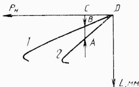
1—диаграмма разрыва пробы ткани; 2— диаграмма разрыва пробы шва; CD — фактическая величина усилия
