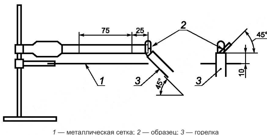
Рисунок 1 — Схема установки для испытания горизонтально закрепленного образца (метод А)
