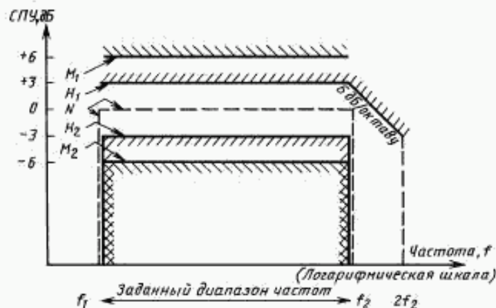
Спектр плотности ускорения (СПУ) и границы допусков
