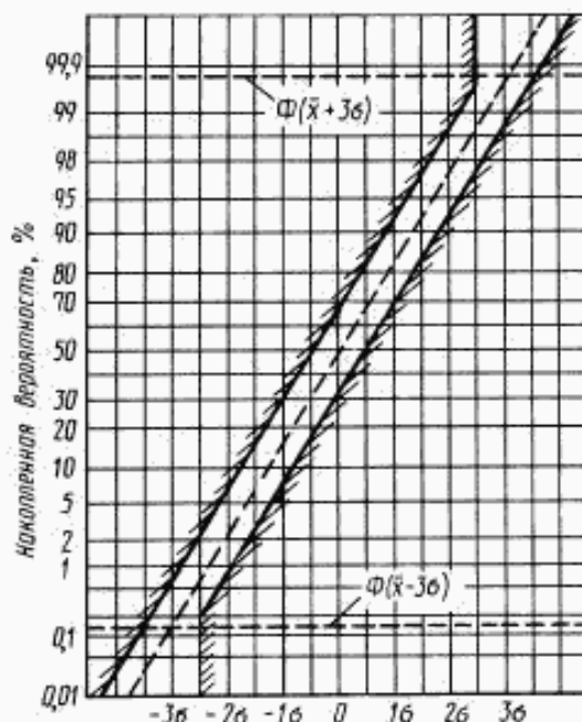
а — кумулятивное среднее квадратическое значение ускорения
