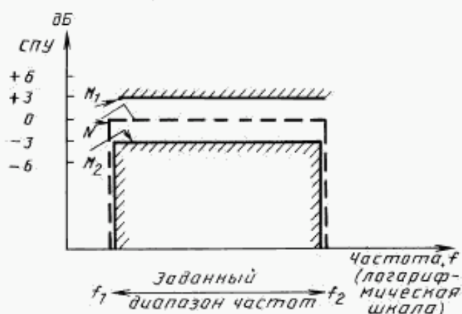
Спектр СПУ и диапазон допусков
