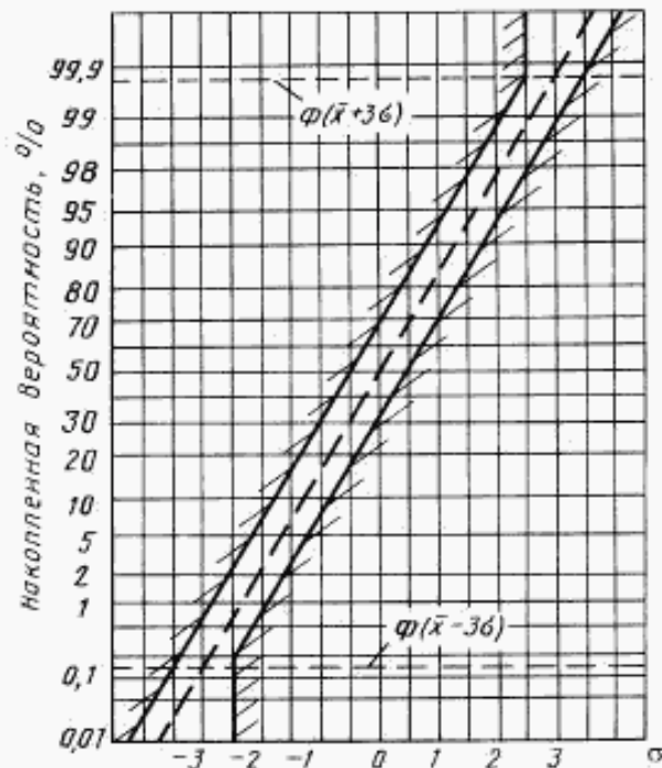
Зона допусков для распределения мгновенных значений ускорения
