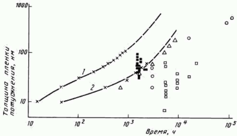
Кинетика потускнения серебра при 75 %-ной относительной влажности по сравнению с данными натуральных испытаний
