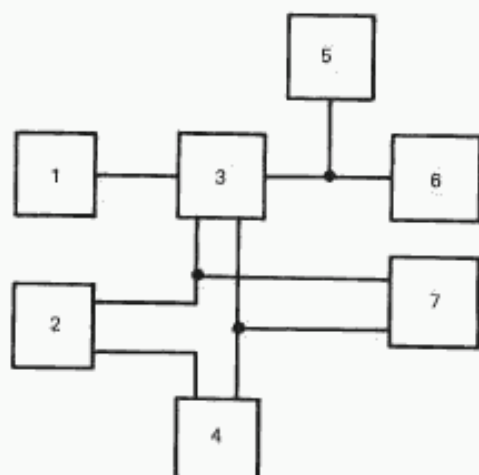
1 — измерительный компакт-диск (п. 2.2.14); 2 — амперметр переменного и постоянного тока (п. 2.2.18); 3 — измеряемый проигрыватель; 4 — автотрансформатор (п. 2.2.17); 5 — эквивалент резистивно-емкостной нагрузки (п. 2.2.15); 6 — вольтметр В2 (п. 2.2.4); 7 — вольтметр переменного и постоянного тока (п. 2.2.19)
