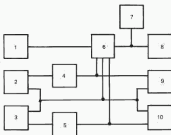
1 — измерительный компакт-диск (п. 2.2.14); 2, 3 — источник постоянного тока (п. 2.2.20); 4, 5 — амперметр переменного и постоянного тока (п. 2.2.18); 6 — измеряемый проигрыватель; 7 — эквивалент резистивно-емкостной нагрузки (п. 2.2.15); 8 — вольтметр В2 (п. 2.2.4); 9, 10 — вольтметр В3 (п. 2.2.19)
