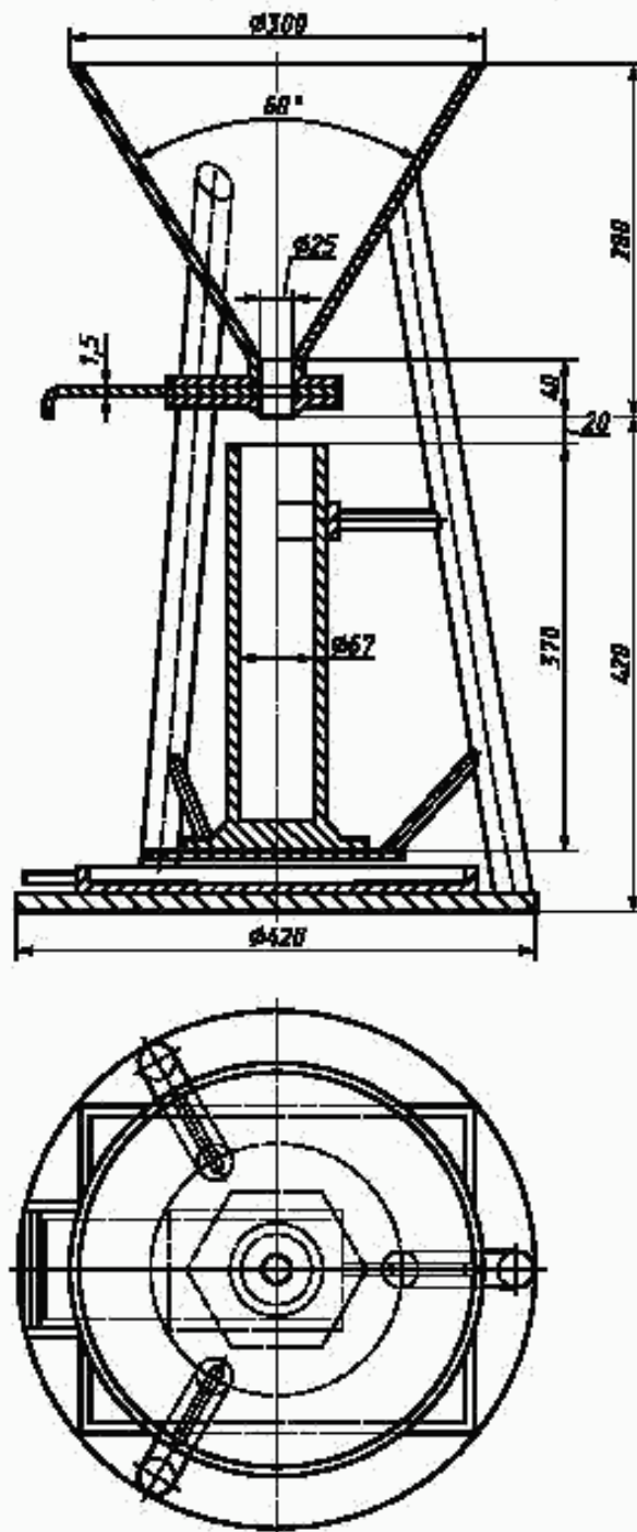
Аппарат для определения насыпной плотности удобрений
