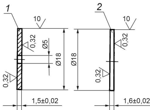
1 — шаблон № 1; 2 — шаблон № 2
