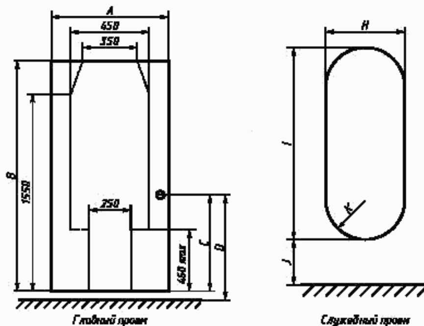
Рисунок 4 — Проемы кабин
