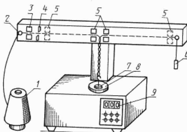
Схема прибора ПОН
