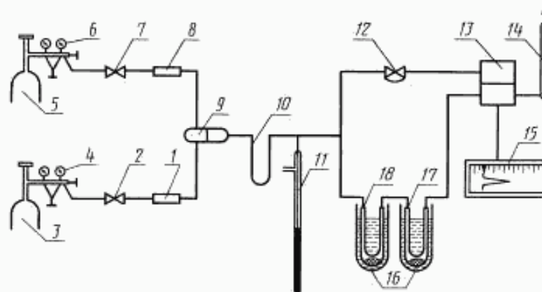
Схема установки для измерения удельной поверхности
