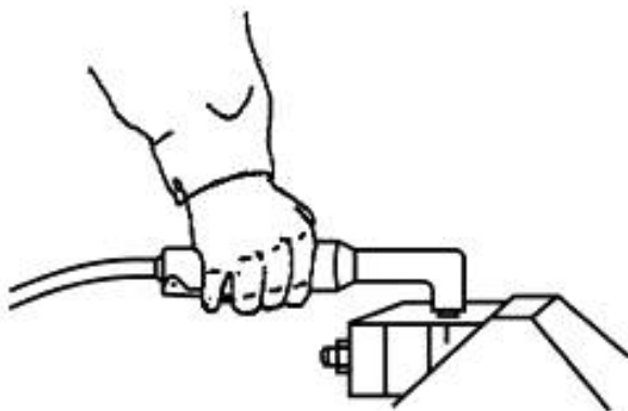
Рисунок 21 — Рабочая поза оператора при испытании машины с прямой основной рукояткой и угловой головкой (см. рисунок 5)
