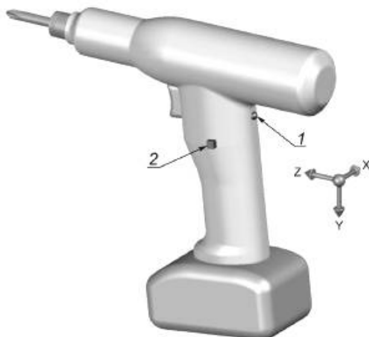
Рисунок 20 — Точки и направления измерений для шуруповерта с центрированной рукояткой пистолетного типа
