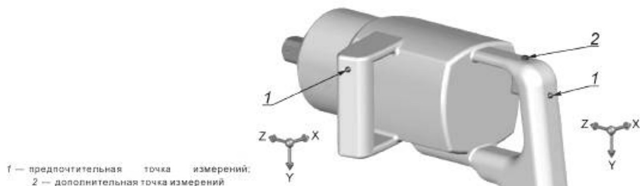
Рисунок 13 — Точки и направления измерений для ударного/импульсного гайковерта с дугообразными основной и поддерживающей рукоятками
