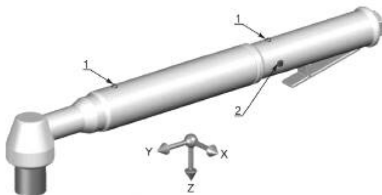
Рисунок 16 — Точки и направления измерений для углового гайковерта
