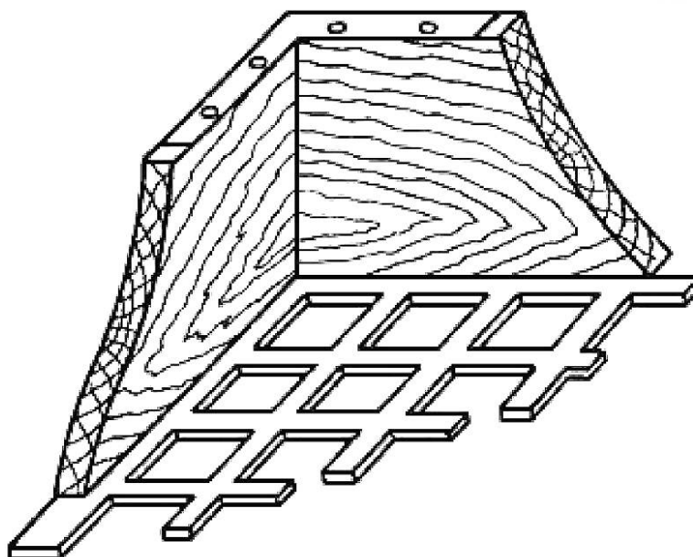
Рисунок 2 — Деталь сита
