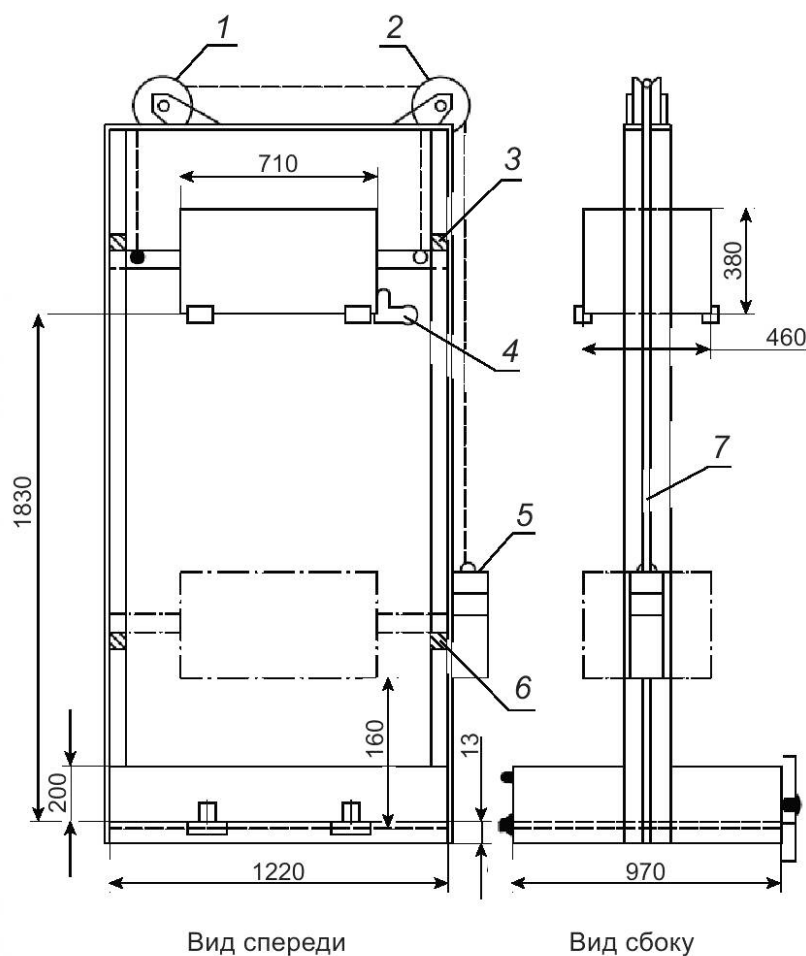
1 — одинарный шкив; 2 — двойной шкив; 3, 6 — стопоры; 4 — защелка; 5 — противовес; 7 — направляющий паз
