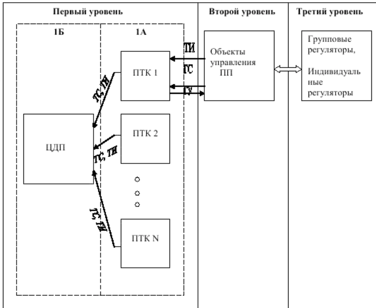
Структура АСУ освещением дорог
