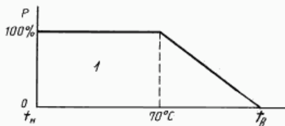
I — рекомендуемая зона эксплуатации; t_n — нижняя температура категории; t_\theta — верхняя температура категории
