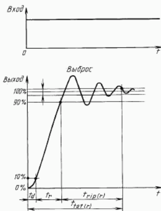
Времена переходного процесса
