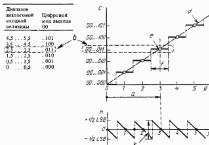
а) Идеальный линейный АЦП
