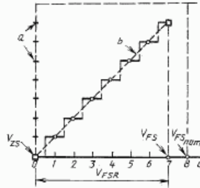
а) Однополярный АЦП
