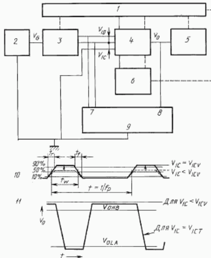
Измерение пускового синфазного входного напряжения
