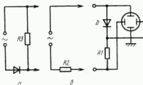
Схема измерения обратного тока (метод осциллографа)
