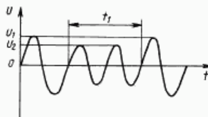
Форма сигнала провала переменного напряжения
