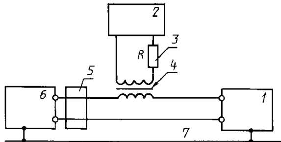
I — испытуемое изделие; 2 — генератор; 3 — сопротивление связи, R = 40 Ом; 4 — соединительный трансформатор; 5 — дополнительное средство защиты от помех; 6 — внешнее устройство; 7 — опорная земля
