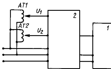
I — испытуемое изделие; 2 — имитатор помех; AT1 , AT2 — автотрансформаторы
