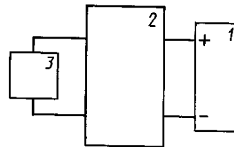
I — испытуемое изделие; 2 — имитатор помех; 3 — блок питания
