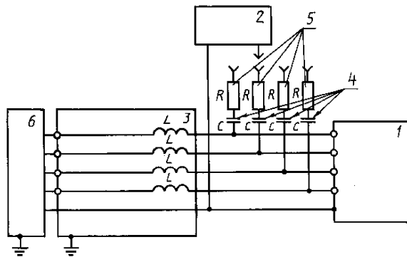
I — испытуемое изделие; 2 — генератор; 3 — разделительное устройство, L = 1,5 мГн; 4 — конденсатор связи, C = 0,5 мкФ (4 шт.); 5 — сопротивление связи, R = 40 Ом (4 шт.); 6 — внешнее устройство
