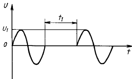
Форма сигнала прерывания переменного напряжения
