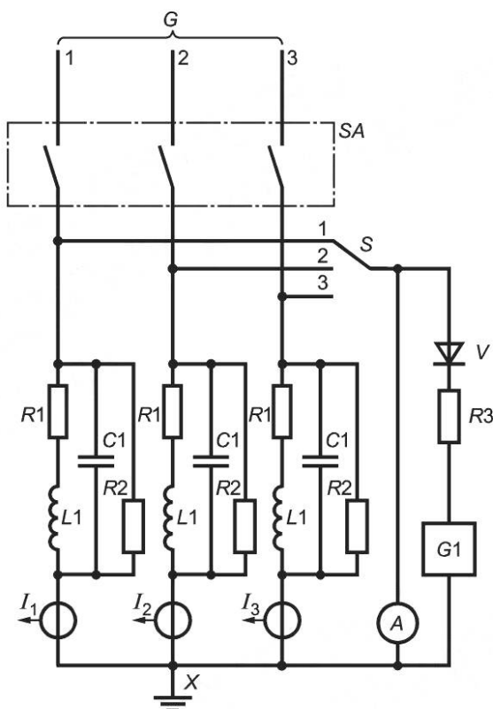
Схема способа регулировки цепи нагрузки
