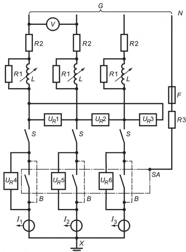
Схема испытательной цепи для проверки включающей и отключающей способности трехполюсного аппарата
