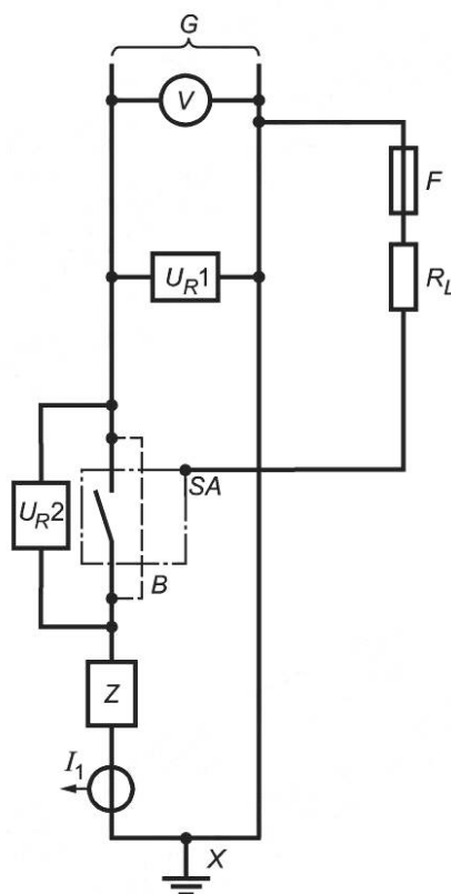
Схема испытательной цепи для проверки включающей и отключающей способности однополюсного аппарата при однофазном переменном или постоянном токе
