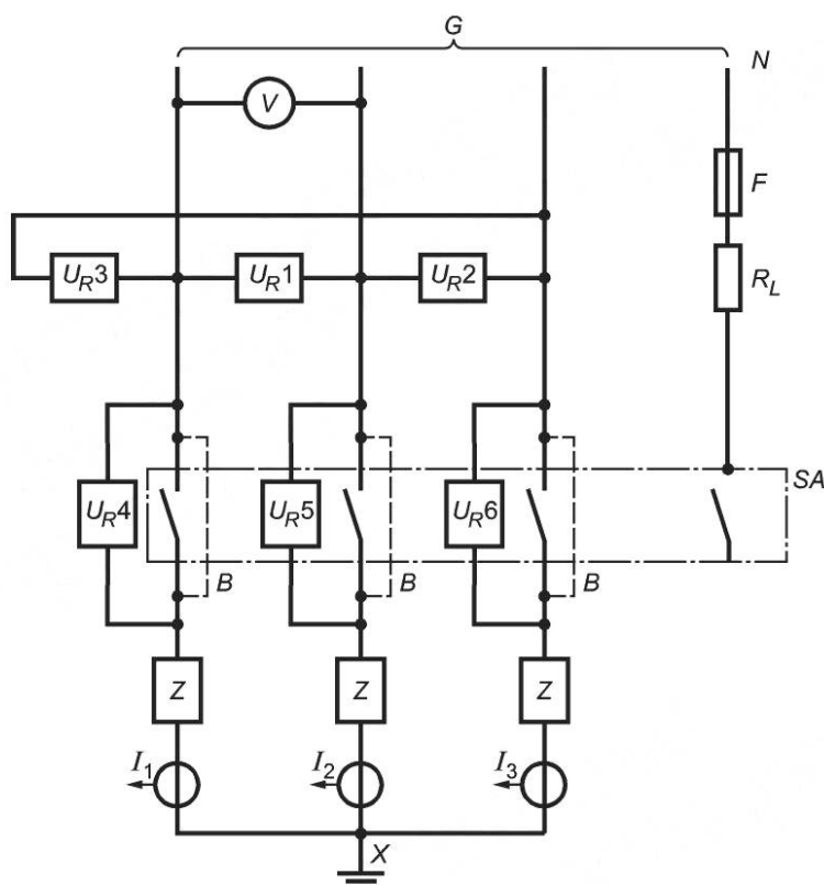
Схема испытательной цепи для проверки включающей и отключающей способности четырехполюсного аппарата
