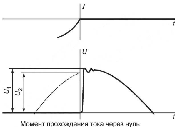
Чертеж 6
