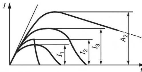
Чертеж 13
