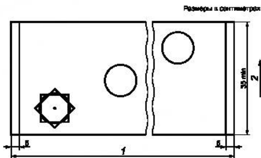
Рисунок 1 — Предлагаемый метод вырезания образцов
