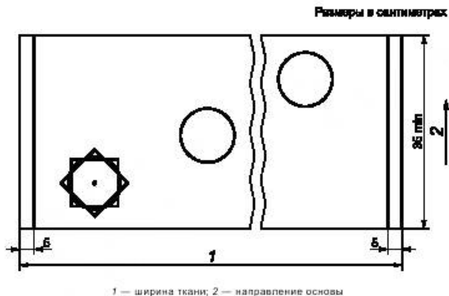
Рисунок 2 — Метод отбора образцов для ткани шириной более 50 см
