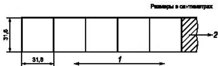
Рисунок 1 — Метод отбора образцов для матов
