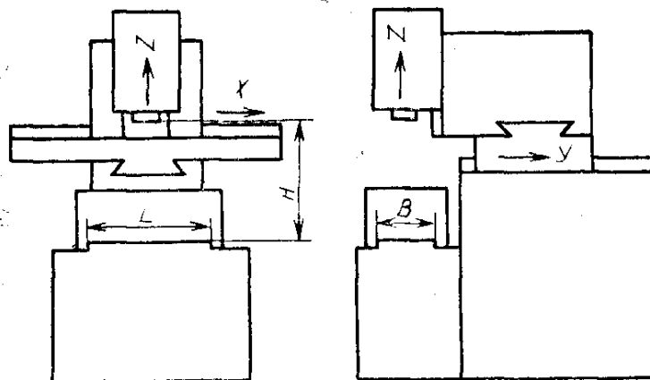
Станок с неподвижным столом
