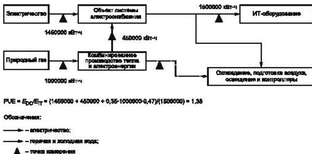
Рисунок В.6 — Метод 2. Расчет на основе энергии, необходимой для производства холодной воды
