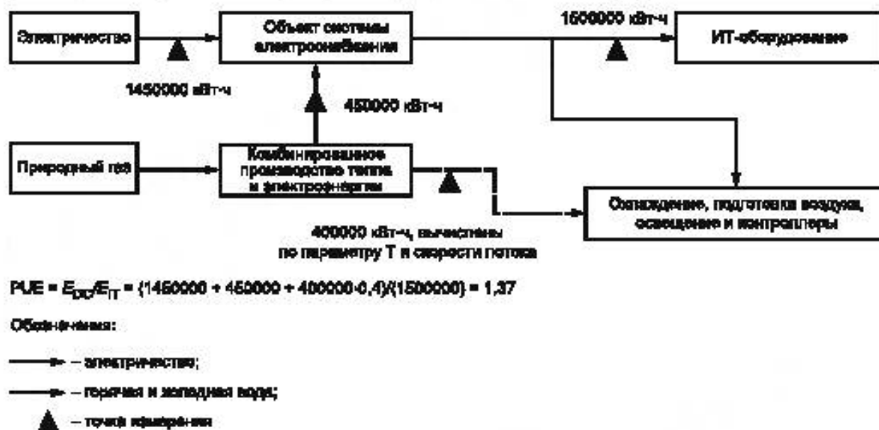
Рисунок В.5 — Метод 1. Измерение по скорости потока холодной воды
