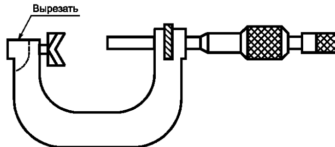
Рисунок В.2 — Микрометр для измерений
