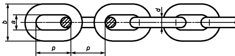
Рисунок 1 — Калиброванная цепь
