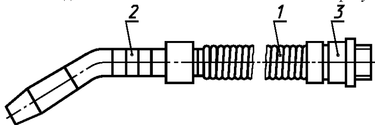
1 — рукав; 2 — наконечник; 3 — патрубок
