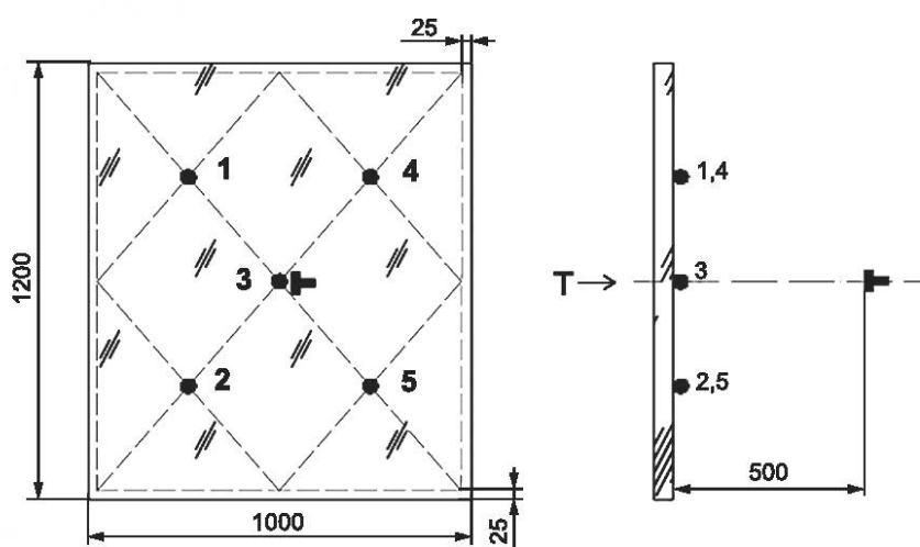
Рисунок А.1 — Пример установки образца в ограждающую конструкцию
