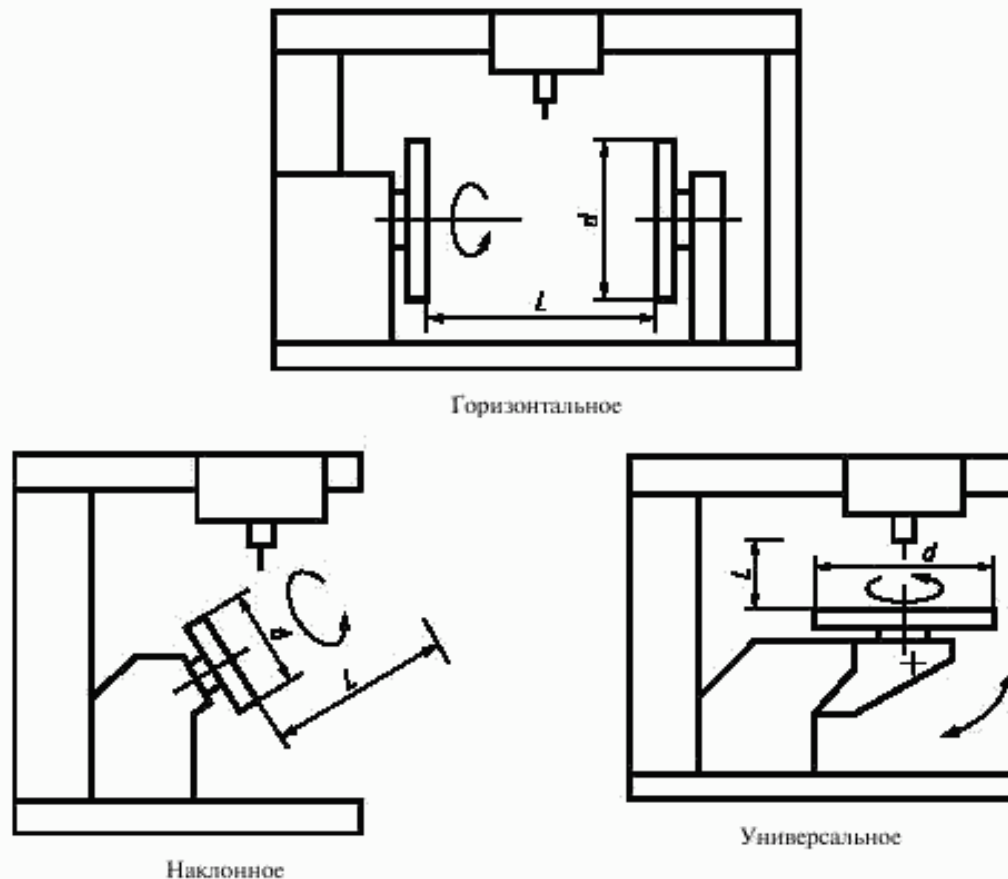
d — наибольший диаметр наплавляемой поверхности; L — наибольшая длина наплавляемого изделия Рисунок 1 — Исполнения оборудования в зависимости от расположения оси вращения изделия
