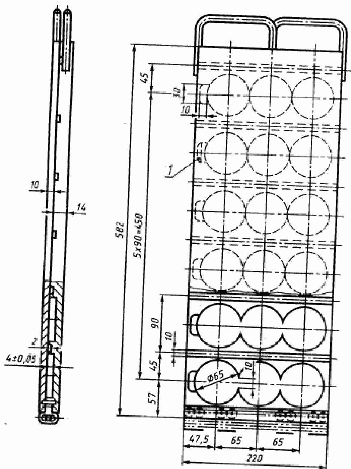
Рисунок 2 — Пресс-форма для вулканизации образцов в виде дисков
