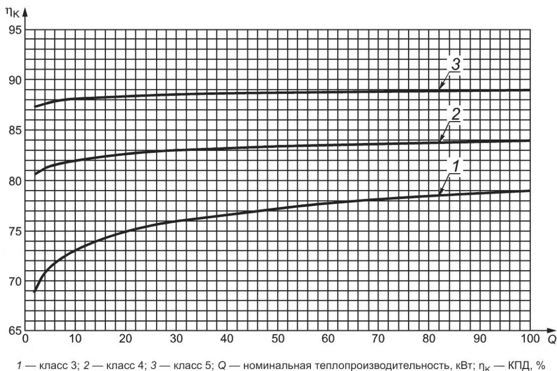
Рисунок 1 — КПД котла
