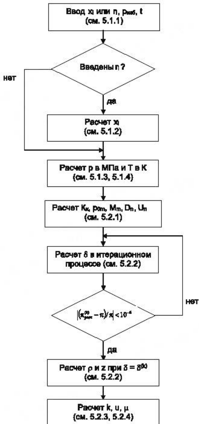
Рисунок 1 — Блок-схема расчета физических свойств природного газа
