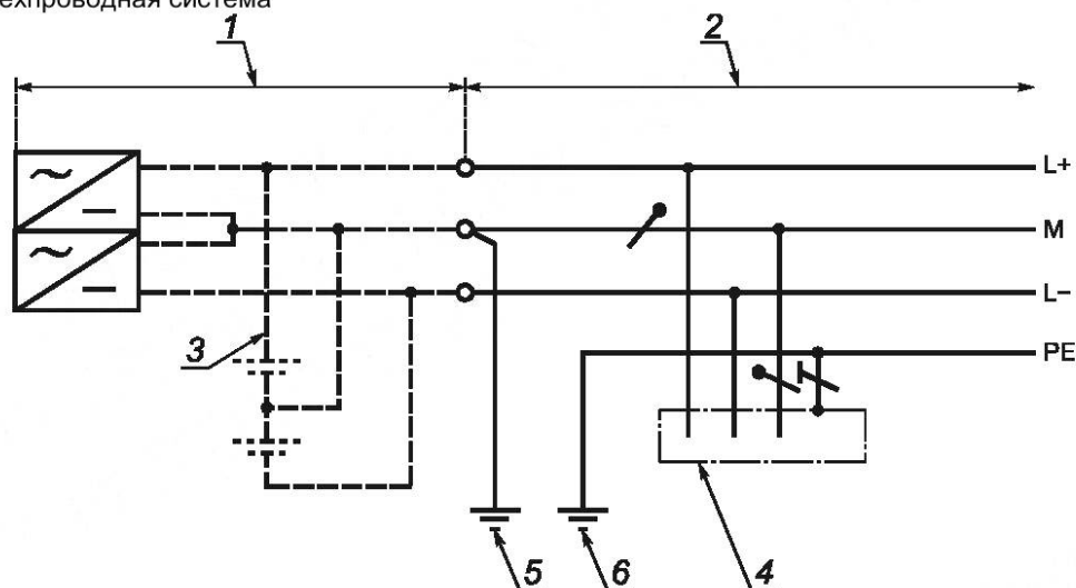
Тип б) – трехпроводная система
