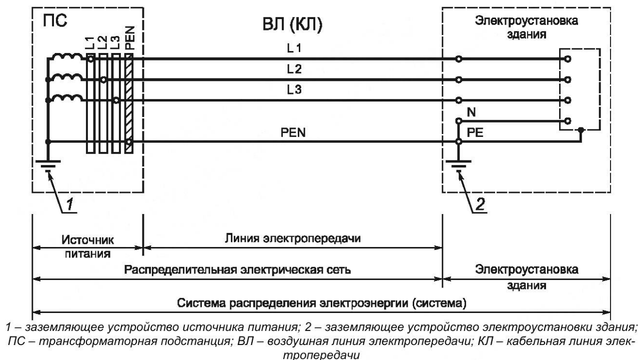
Рисунок 20.2 – Общий вид системы распределения электроэнергии
