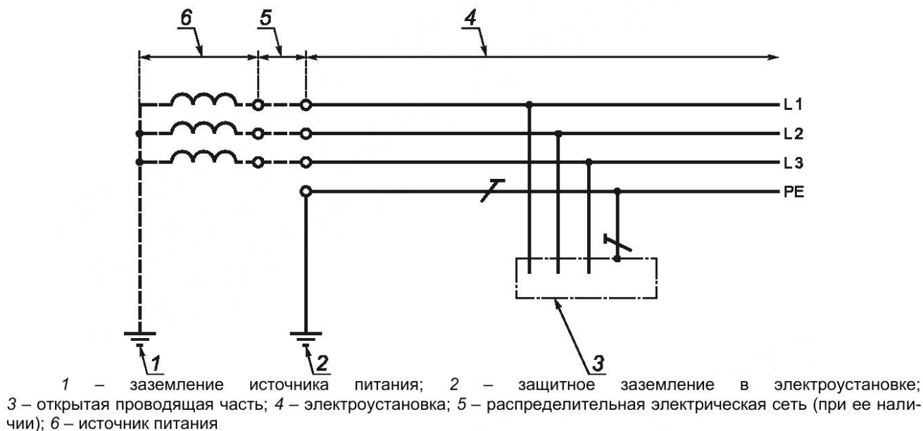
Рисунок 31F1 – Система TT трехфазная четырехпроводная с заземленным защитным проводником и нейтральным проводником во всей системе
