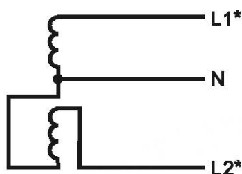
Рисунок 1 – Однофазная двухпроводная электрическая цепь
