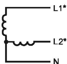
Рисунок 2 – Однофазная трехпроводная электрическая цепь
