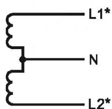
Рисунок 2 – Однофазная трехпроводная электрическая цепь
