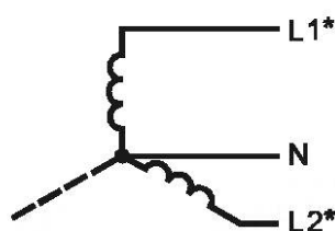
Рисунок 2 – Однофазная трехпроводная электрическая цепь
