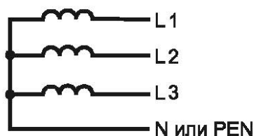
Рисунок 5 – Трехфазная четырехпроводная электрическая цепь
