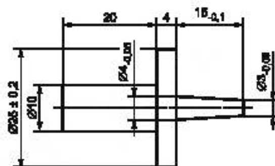
Рисунок 2 – Испытуемый стержень
