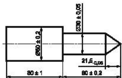
Рисунок 3 – Испытуемый щуп
