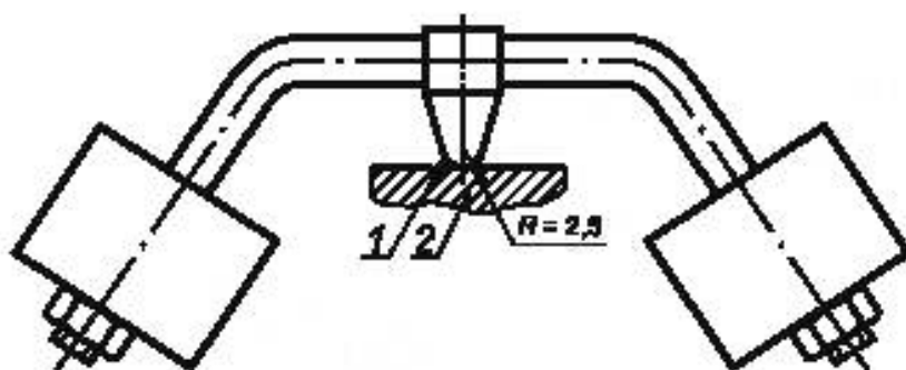
Рисунок 12 – Устройство для вдавливания шарика
