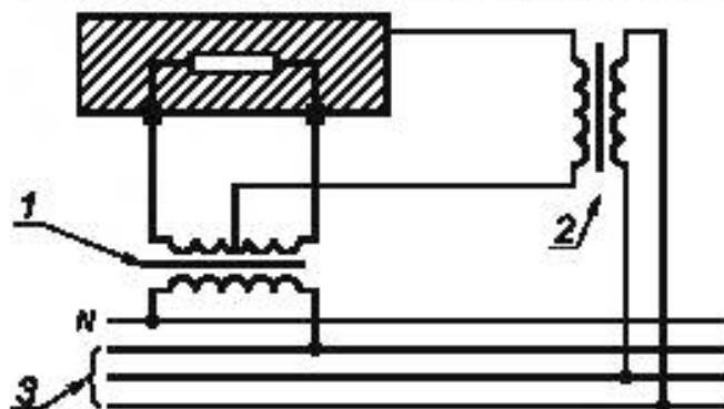
1 – разделительный трансформатор; 2 – повышающий трансформатор; 3 – трехфазная сеть
