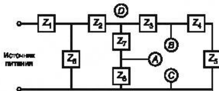
D – наиболее удаленная от источника питания точка, в которой мощность, подаваемая на внешнюю нагрузку, превышает 15 Вт; A и B – наиболее близкие к источнику питания точки, в которых мощность, подаваемая на внешнюю нагрузку, не превышает 15 Вт. Это маломощные точки. Точки A и B раздельно накоротко соединены с точкой C. Условия повреждения а) – ф) по 20.11.2 рассматриваются в каждой из цепей Z 1 , Z 2 , Z 3 , Z 6 и Z 7 при необходимости
