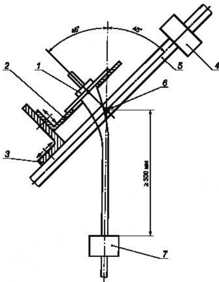
1 – образец; 2 – регулируемая несущая плата; 3 – регулируемый хвостик; 4 – противовес; 5 – качающаяся рама; 6 – ось качения; 7 – груз
