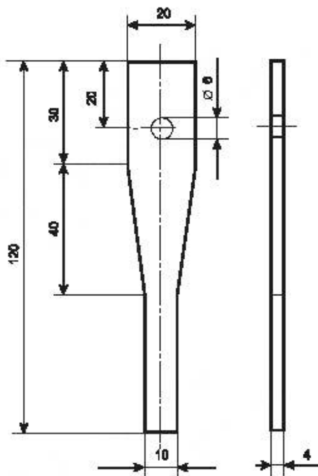
Рисунок R.3 – Стальная пружина
